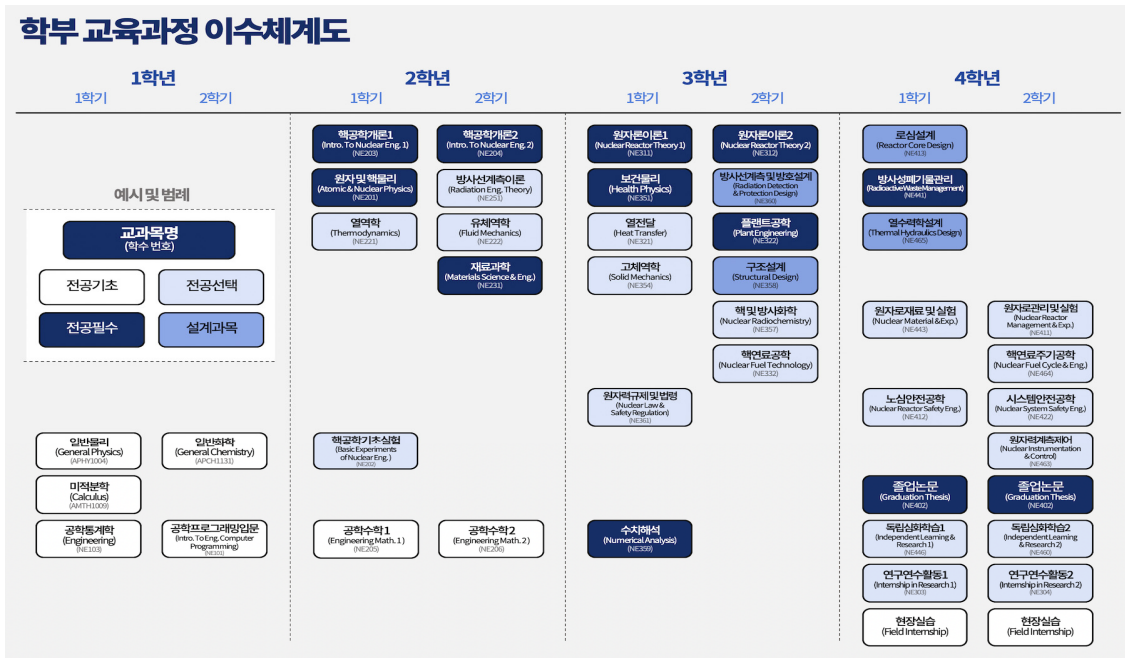
[교육과정 체계도]
